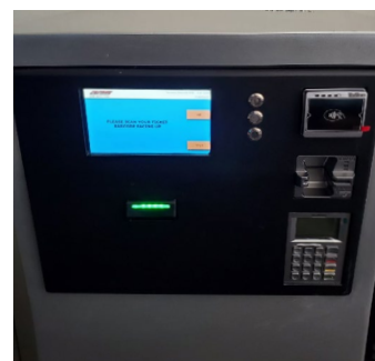
Interfaccia del parking kiosk con PP54 Evo installata
