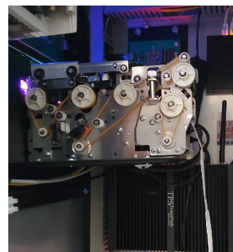
PP54 EVO - vista interna del parking kiosk
